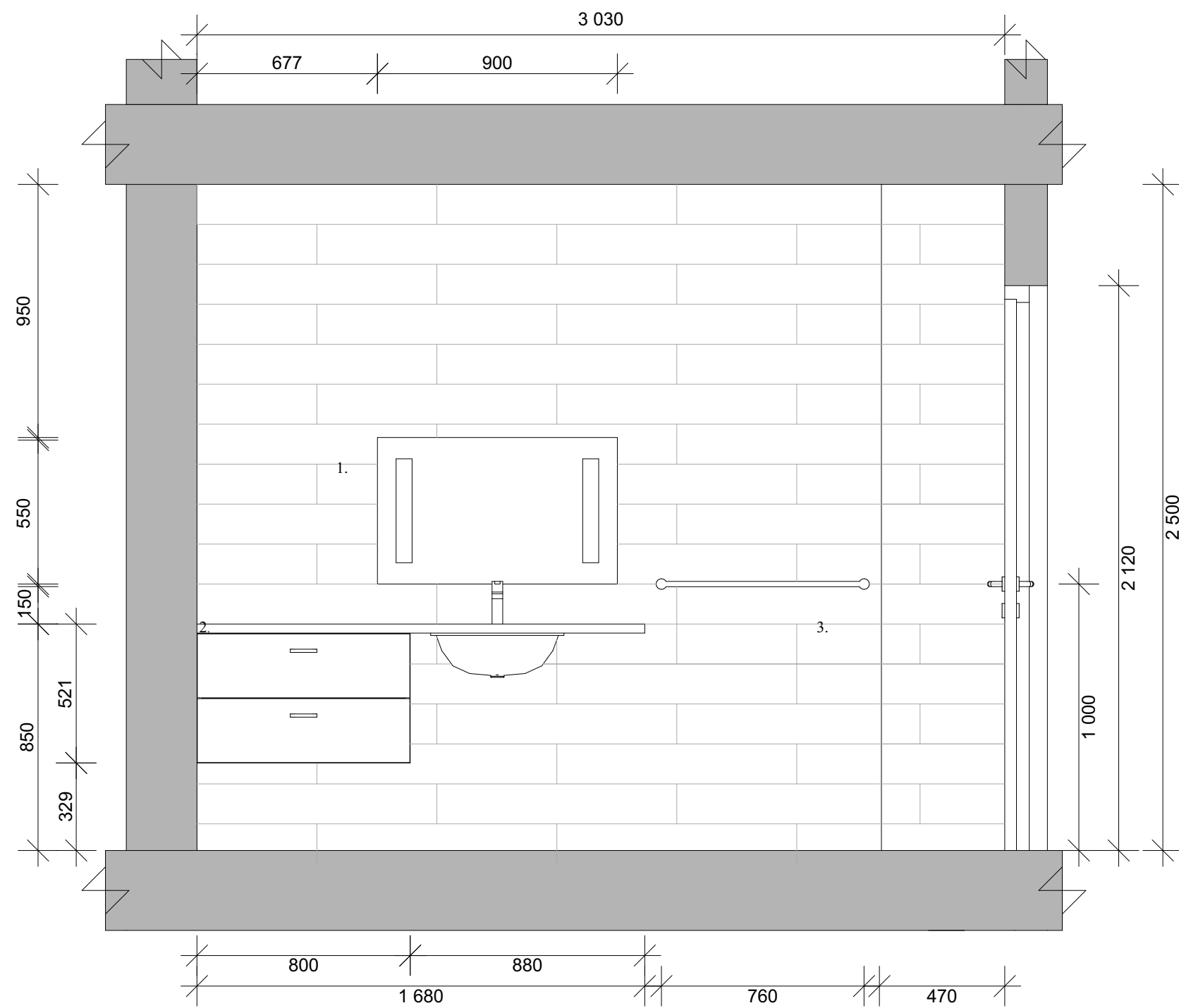
Snitt A
