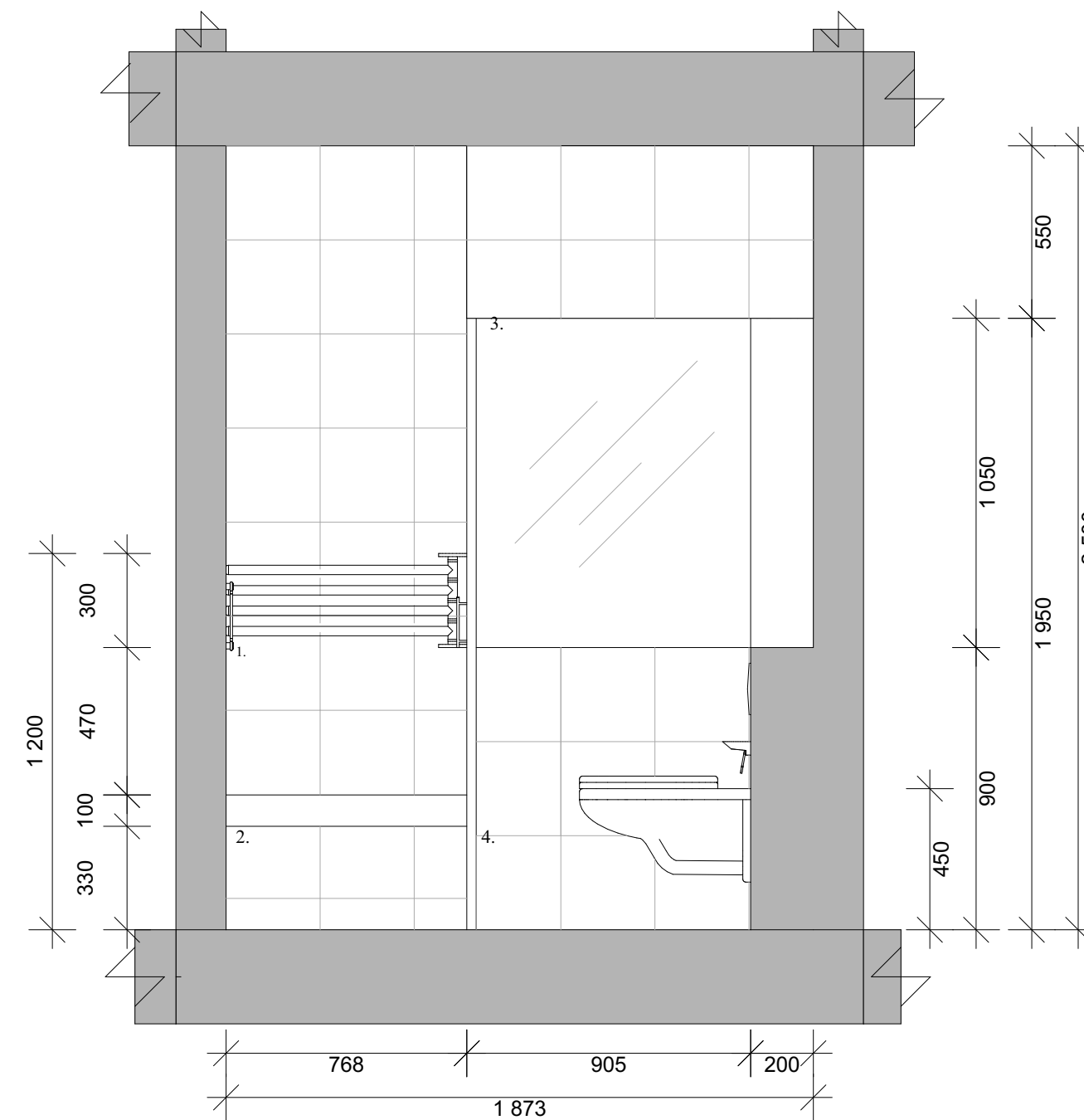
Snitt C
