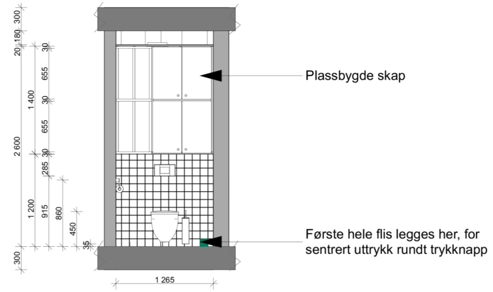
Snitt A:A
