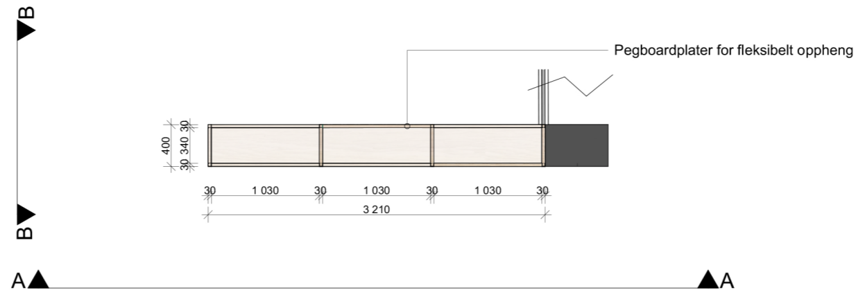
Plan (utsnitt)
