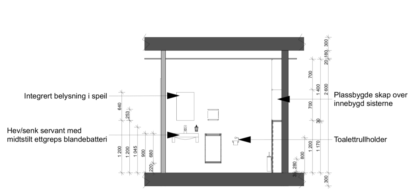
Snitt D:D
