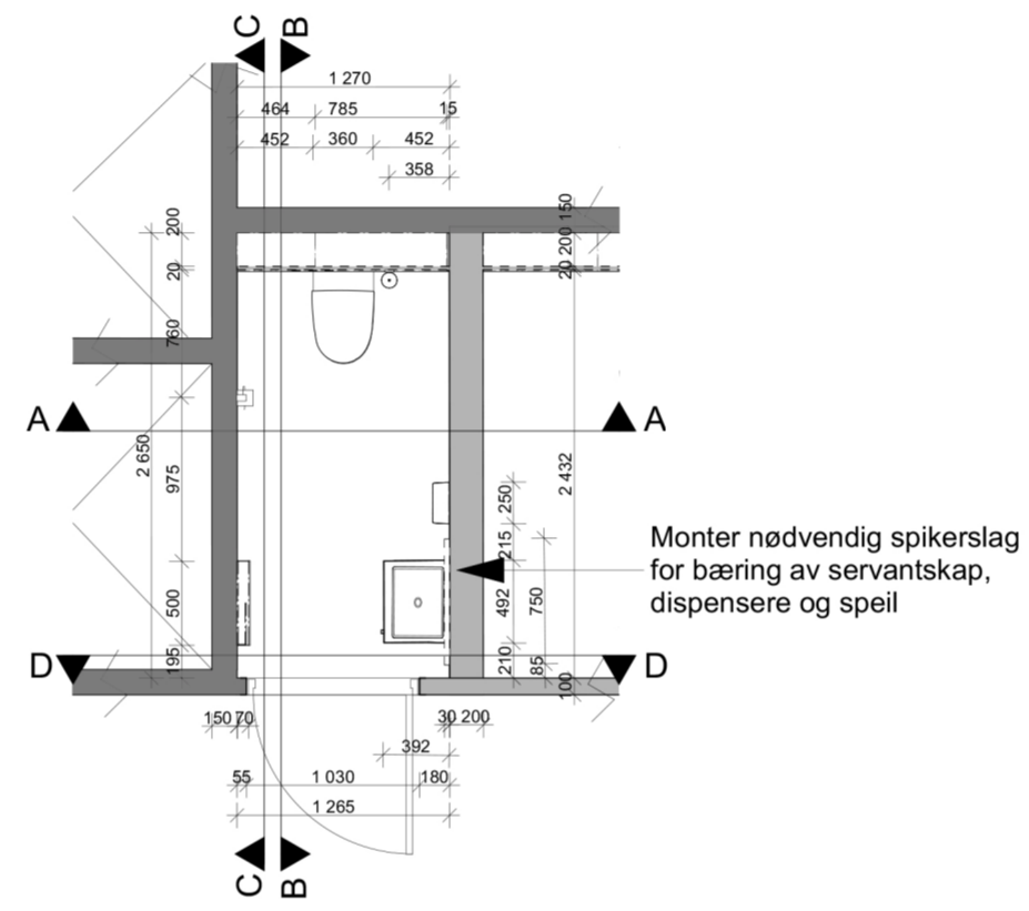
Plan (utsnitt)
