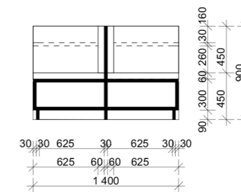
Snitt A:A 1:50
