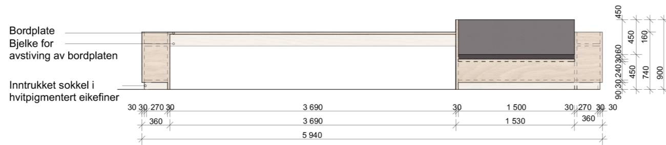
Oppriss A
