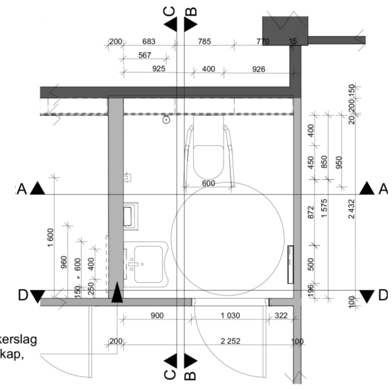
Plan (utsnitt)
