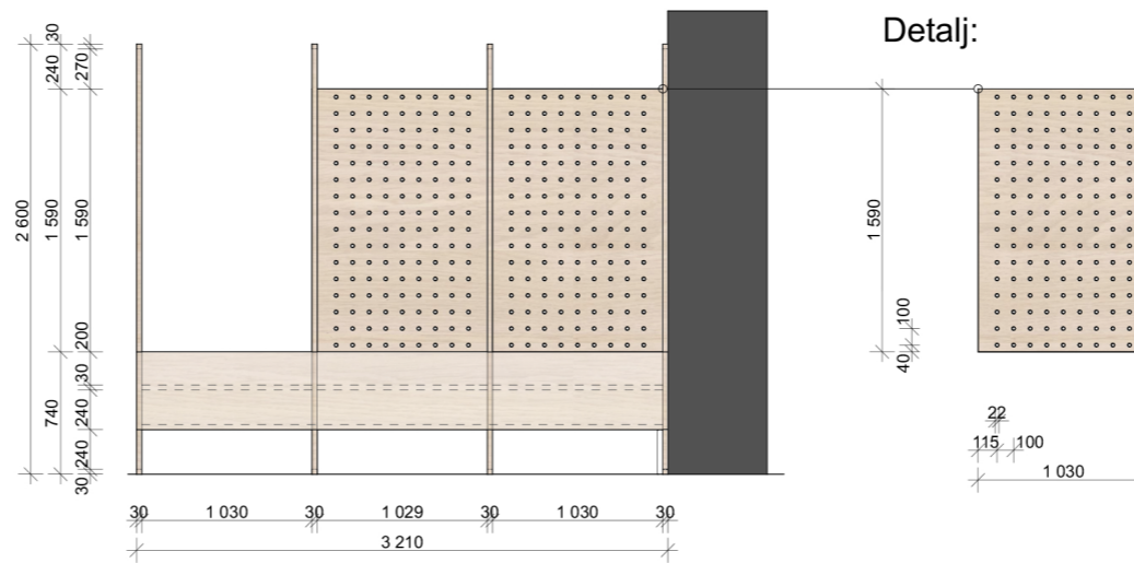
Oppriss A
