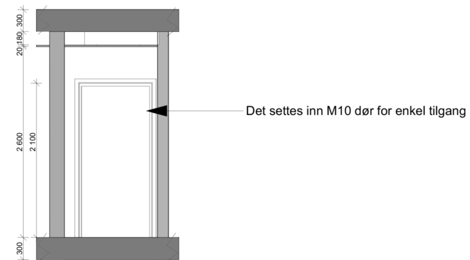
Snitt C:C
