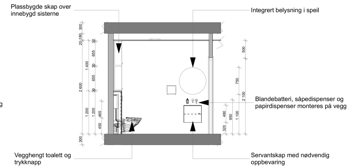
Snitt B:B
