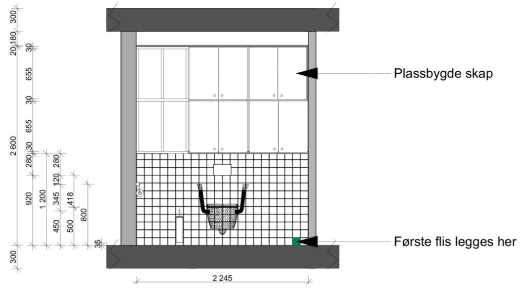
Snitt A:A
