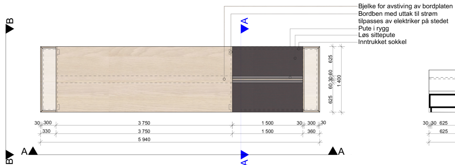
Plan (utsnitt) 1:50
