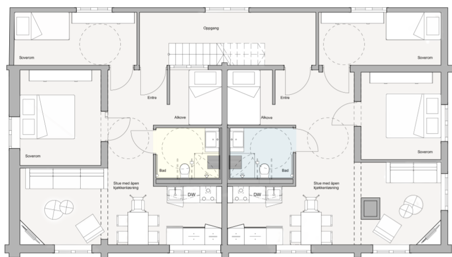
Møbleringsplan: Hovedbygg, 2. etasje
